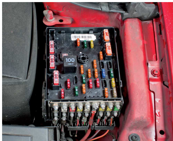
Figura 1: il fusibile del sistema mecatronico si trova solitamente nel portafusibili del vano motore
