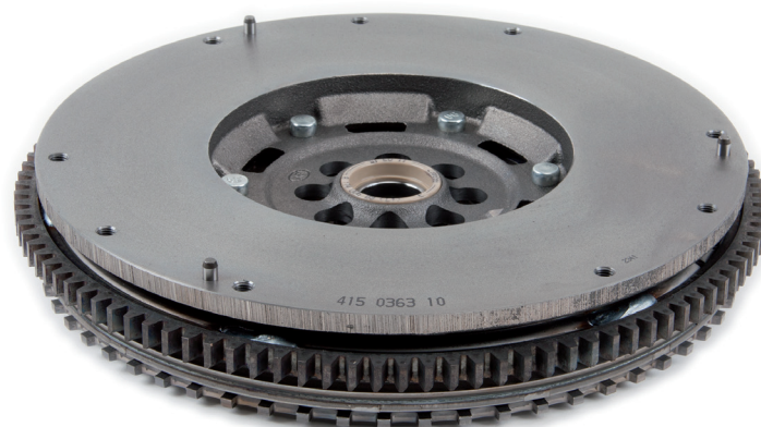
Fig. 1: volano doppia massa LuK 415 0363 11
